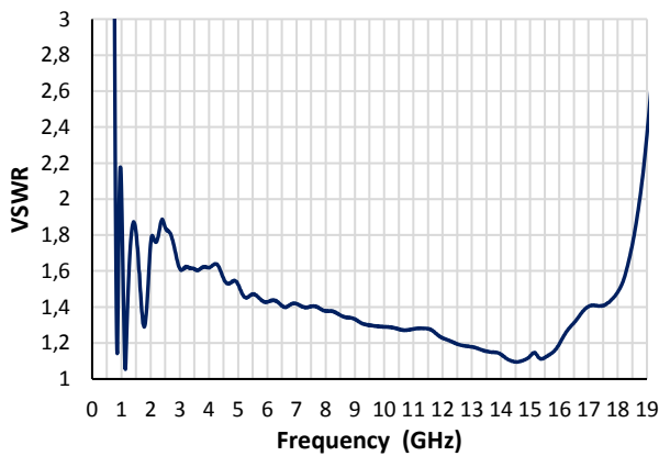
VSWR
